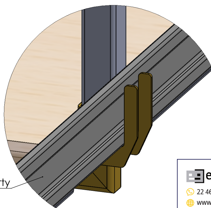
SZCZEGÓŁ C SKALA 1 : 3
