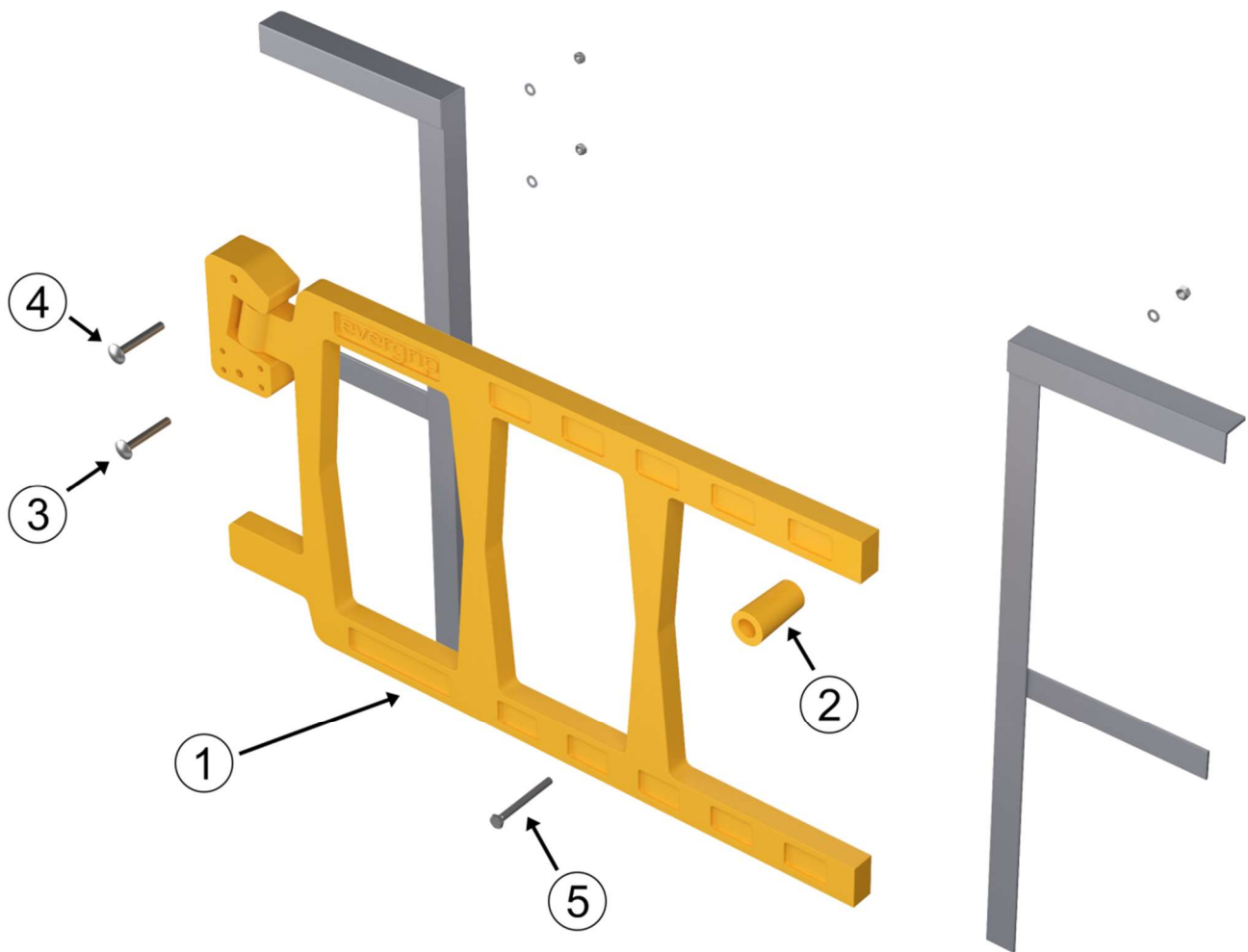
Wykaz elementów stalowych niezbędnych na montażu na kątowniku.
